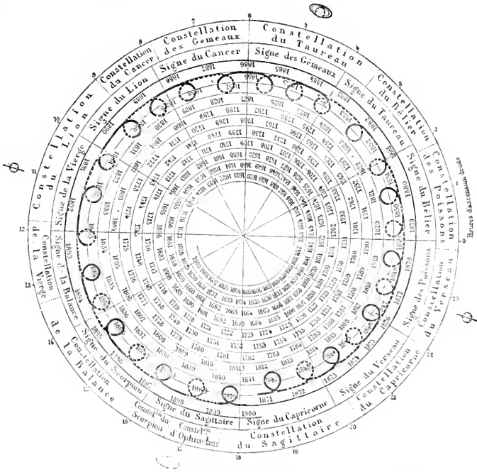
Fig. 281. — Mouvement apparent de Saturne relativement à la Terre et positions dans le z. l. de 1600 à 1900.
