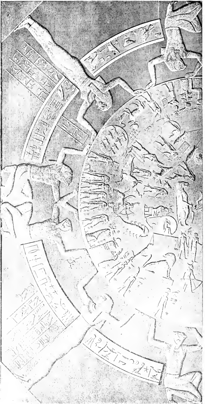
Fig. 239. — ZODIAQUE DE DENDÉRAH : Balance. — Scorpion. — Sagittaire. — Capricorne. — Verseau. — Poissons
