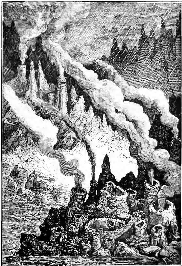
Les geyser de l'Islande donnent peut-être une idée de ce qui se passait au volcan de Linné.
