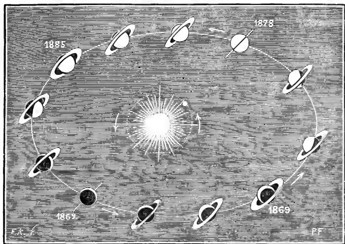
Fig. 203. — Perspective variable des anneaux de Saturne vus de la Terre.
