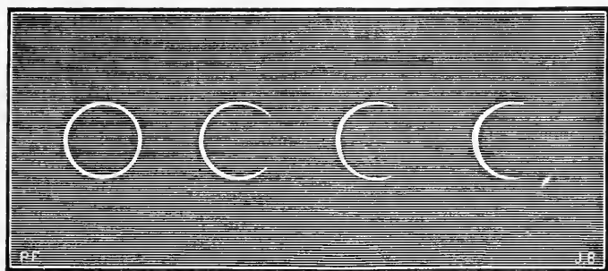
Fig. 140. — Vénus vue sous la forme d'un anneau lumineux
