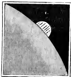
Fig. 217. — Occultation de Jupiter par la Lune, le 24 mai 1860.
