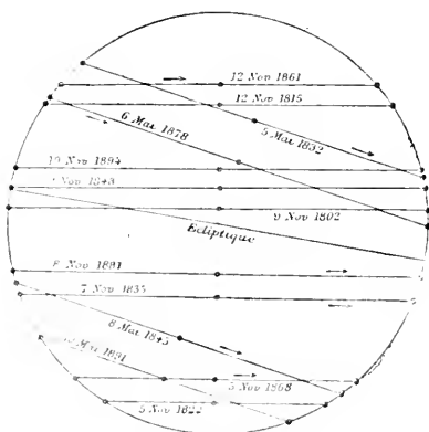
Fig. 143. — Passages de Mercure devant le Soleil pendant le XIX e siècle.
