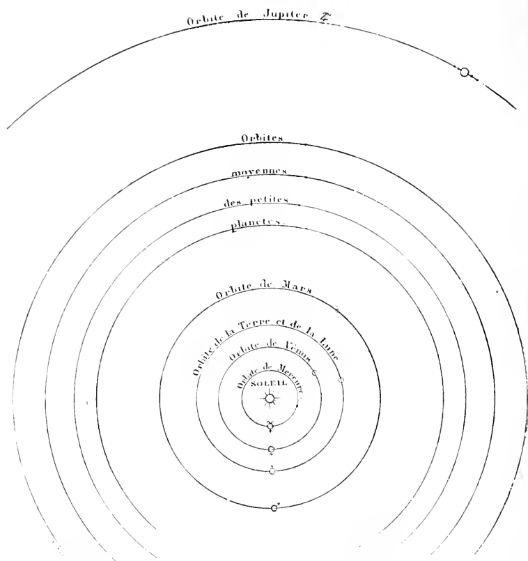
FIG. 179 — Orbite de la Terre et des planètes voisines. (Echelle 1mm = 2 millions de lieues).
