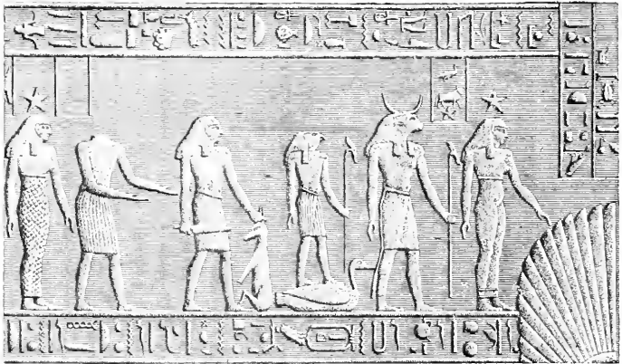
Fig. 272. — Zodiaque de Dendérah. Planètes et constellations
