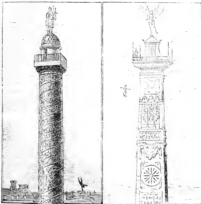
Fig. 17. — Intensité comparée de la pesanteur sur la Terre et sur Mars.
