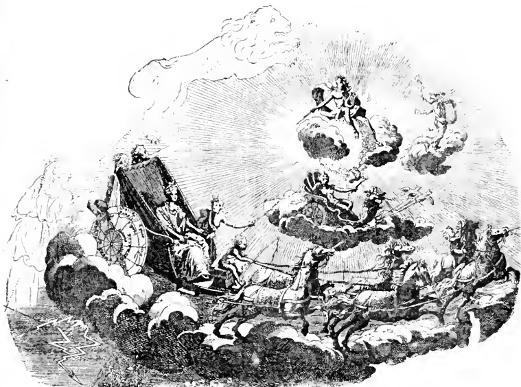
Fig. 105. — La Terre accompagnée de la Lune, Vénus et Mercure, tournant autour du Soleil. (Figure du XVIII e siècle).
