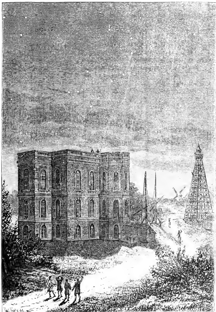
Premières observations de la planète Uranus, le 13 Mars 1781, par Messrs. Lalande & Bode, à l'Observatoire de Paris.
