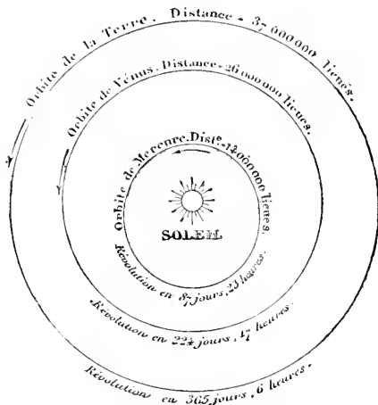
Fig. 151. — Les orbites de Mercure, Vénus et la Terre. Échelle : 1 mm = 1 million de lieues.
