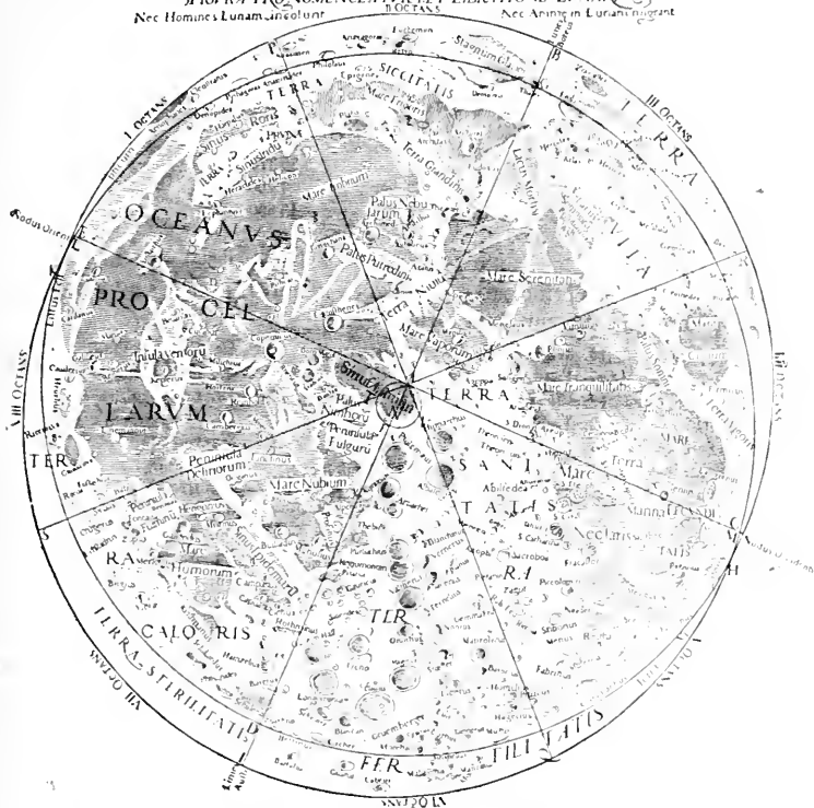
Premières cartes de la Lune: RICCIOLI, 1664
