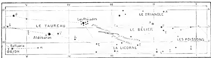
Fig. 290. — Mouvement et positions des planètes Jupiter, Saturne, Uranus et Neptune pendant deux années 1884 et 1886.
