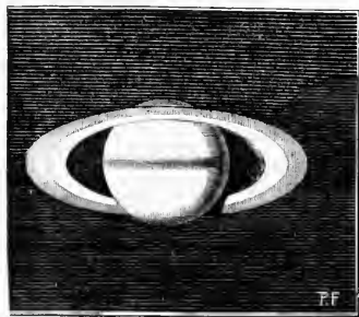
Fig. 290. Premier dessin d'une ligne de séparation entre les anneaux. Cassini 1675.
