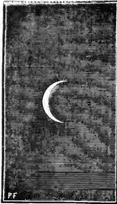
Fig. 113. — La Lune vue à l'œil nu.
