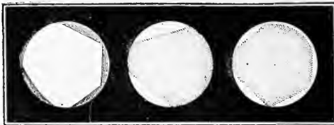
Fig. 267. — Aspects observés sur le IV e satellite de Jupiter.
