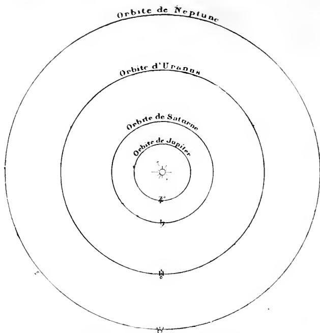
Fig. 320. — Les orbites principales du système solaire.
