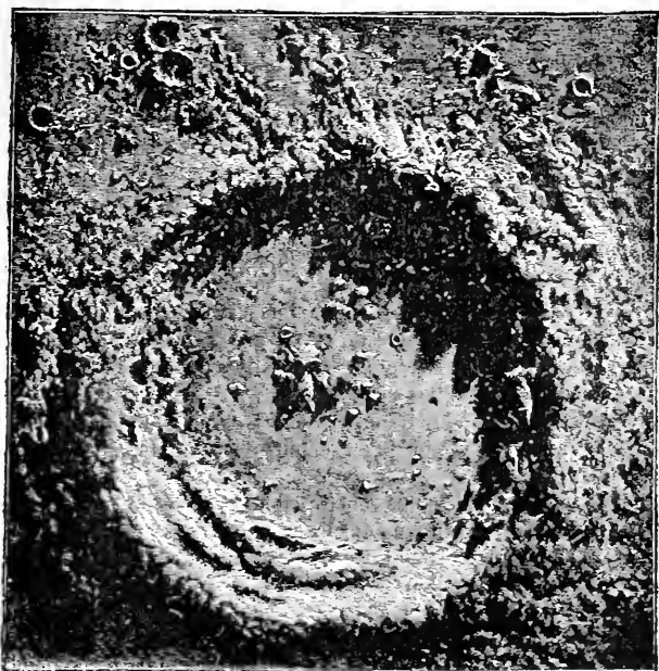
Fig 206. — La montagne lunaire de Copernic. Type des grands cratères.
