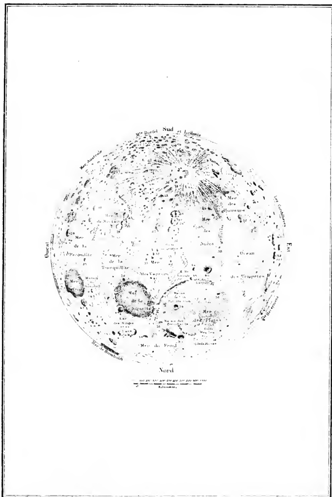
CARTE GEOGRAPHIQUE DE LA LUNE SÉNIÉNOGRAPHIE
