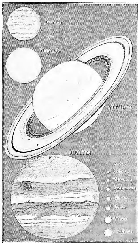
Fig. 263. — Grande et comparaison des différents mondes du système solaire.
