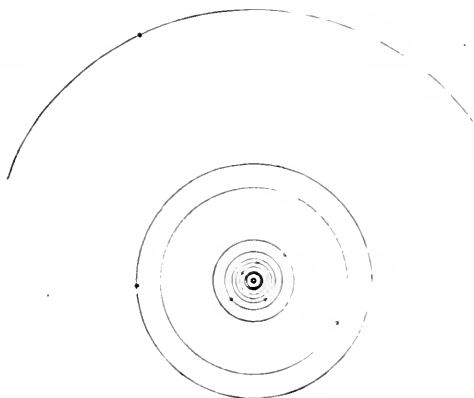
Fig. 300. — Le système de Saturne.
