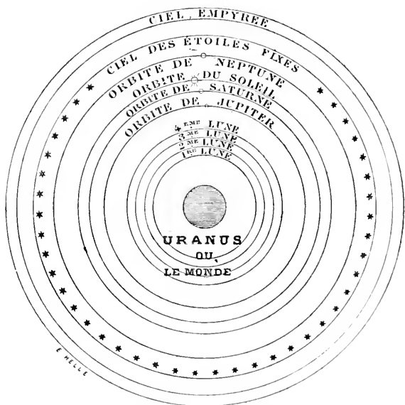
Fig 318. — Le Système du monde pour les habitants d'Uranus.
