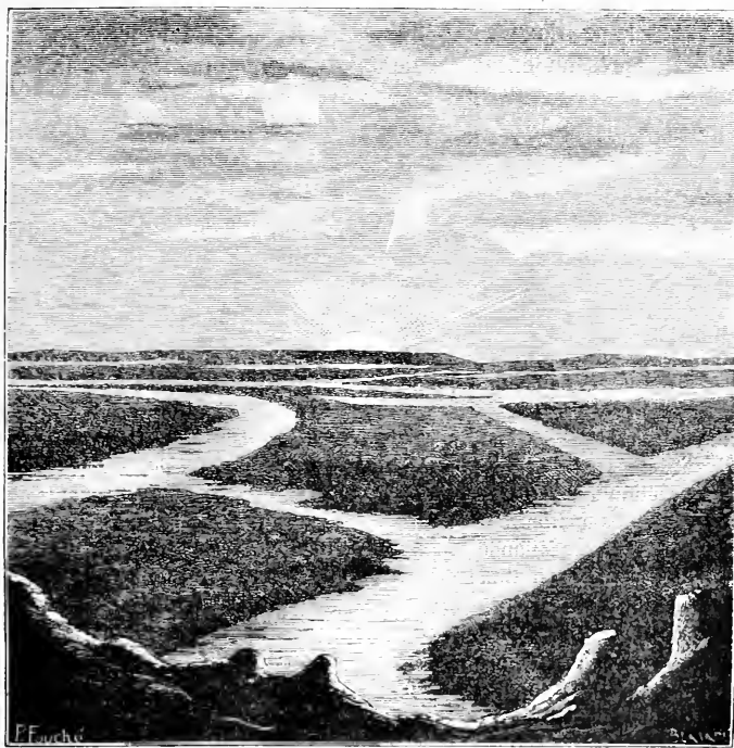
Fig. 34. — Le lever du soleil sur les canaux de Mars.
