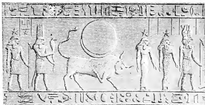
Fig. 275. — Zodiaque de Dendérah. Planètes et constellations — suite
