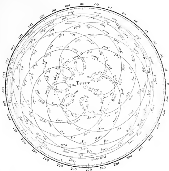
Fig. 11. — Mouvement de Mars par rapport à la Terre.
