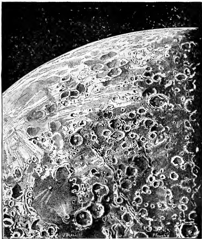
Fig. 201. — Région montagneuse au sud de la mer de la Fécondité.
