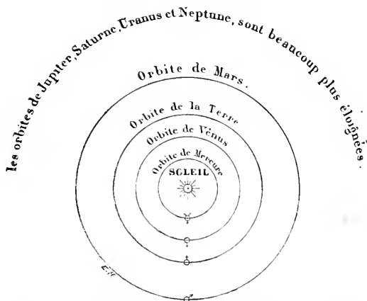
Fig. 8. — Plan du système solaire pour les planètes les plus proches du Soleil. (Échelle : 1 m = 2 millions de lieues.)
