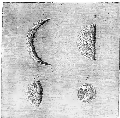
Fig. 117. — Inégalités observées sur la planète Vénus.
