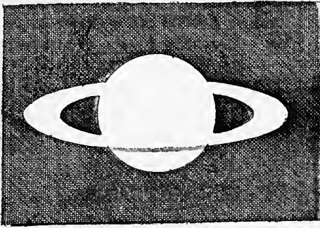
Fig. 288. — Premiers dessins de l'anneau de Saturne. HUYGENS 1659.
