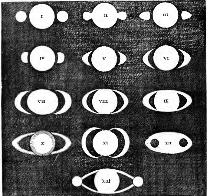
Fig. 285. — Premières représentations de Saturne (1).
