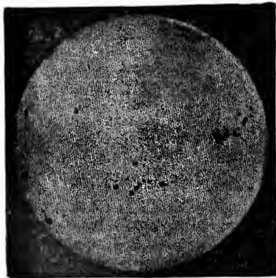
Fig 106. — Aspect des taches solaires.
