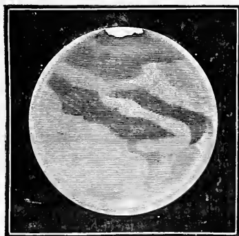
Fig. 59. — Voile atmosphérique sur le contour intérieur de la planète.
