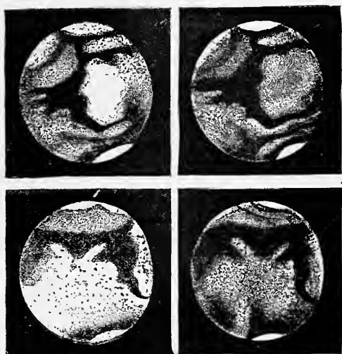
Fig. 13. — Aspects de Mars les 13, 14, 17 et 18 juin 1858.
