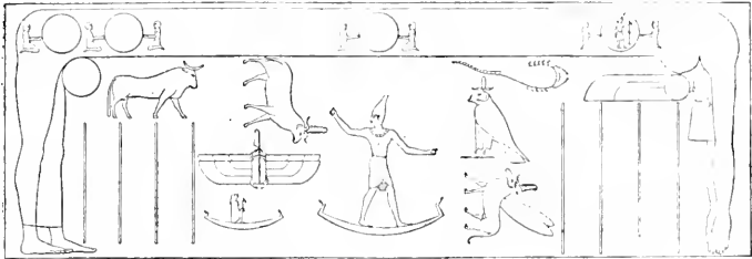
Fig. 277. — Bas-relief astronomique au plafond du temple d'Hermothis.
