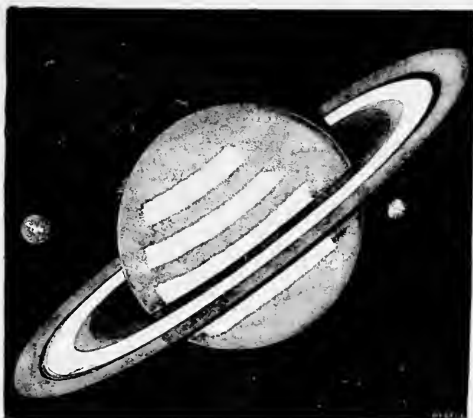
Fig. 282. — Grandeur comparée de Saturne et de la Terre.
