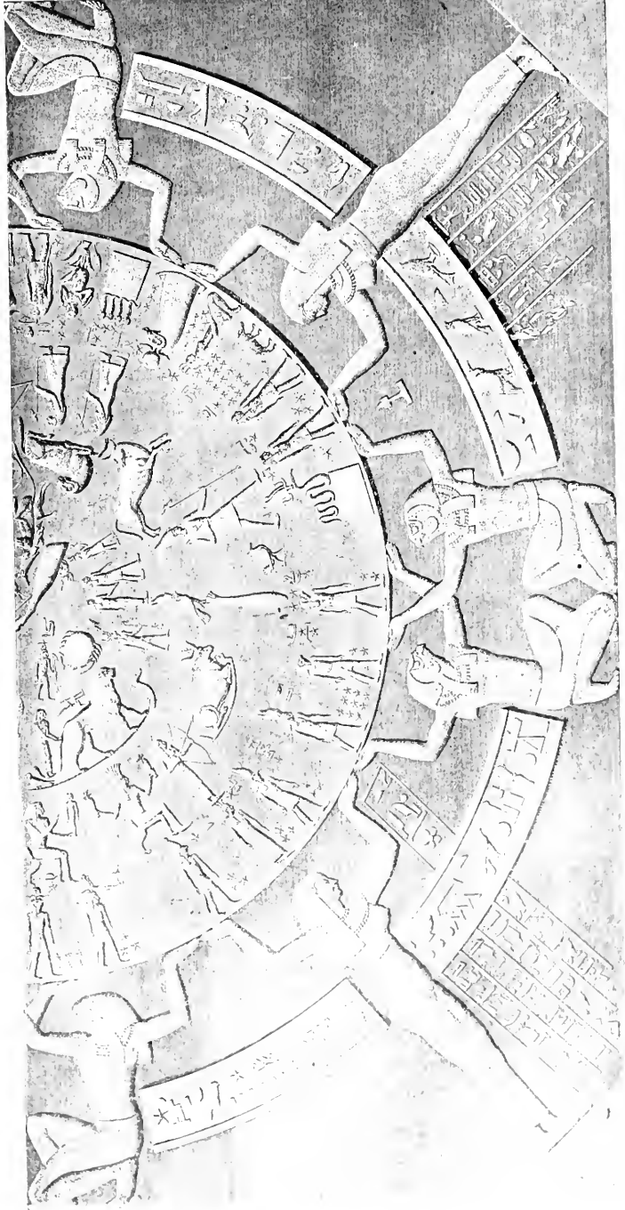
Fig. 230 ZODIAQUE DE DENDÉRAH : Beher — Taucau. — Gemeaux — Cancer. — Lion. — Épi de la Vierge.
