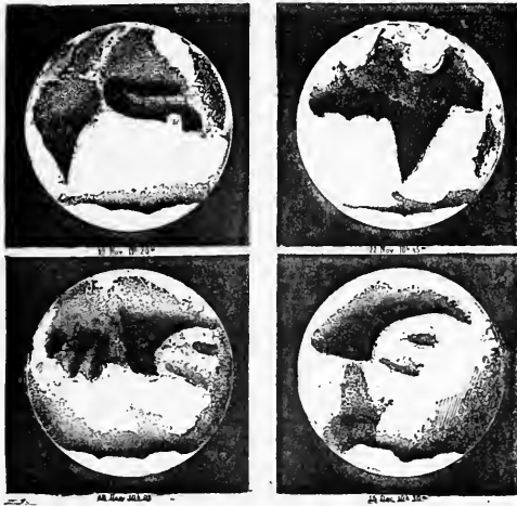
Fig. 15. — Aspects de Mars les 19 et 22 novembre, 18 et 19 décembre 1864.
