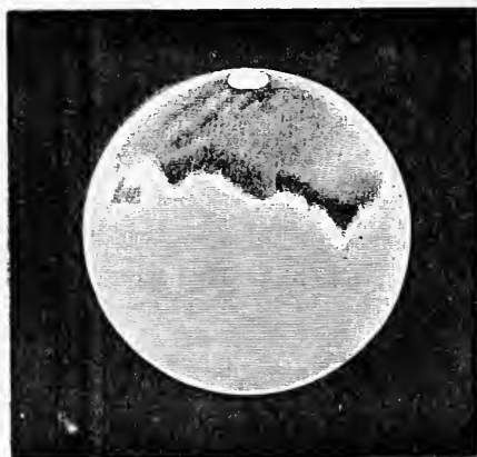
Fig. 63. — Météorologie de Mars — Trainée de nuages le long des côtes.
