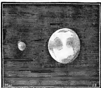
Fig. 119 — Observation problématique du satellite de Venus (Cassini, 1672.)
