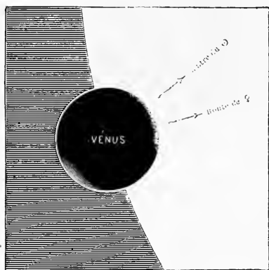
Fig. 15. — L'auréole atmosphérique de Vénus (Allegheny, 6 décembre 1882).
