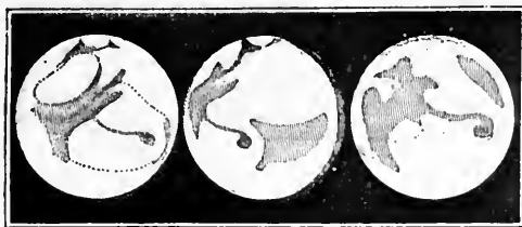
Fig. 11. — Aspects de Mars les 11 septembre et 20 octobre 1830, et le 16 décembre 1832.
