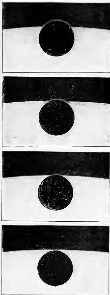
Fig. 139 — L'aurole atmosphérique de Vénus (Postdam, 6 décembre 1882).
