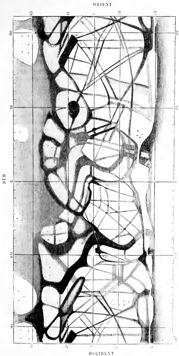
Fig. 30. — Courbes magnétiques observées sur la planète Mars. (Dessin de M. SCHVABILLI) (Aux points signalés par de petits cercles noirs, on a vu des taches blanches comme de la neige.)
