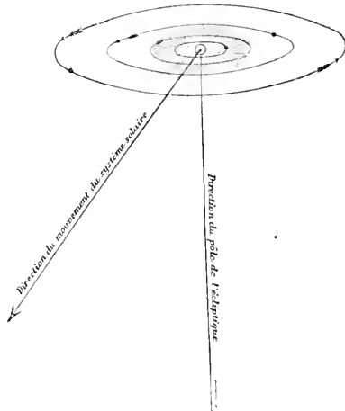
Fig. 184. — Chute du système solaire dans l'espace.
