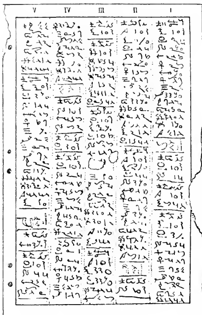
Fig. 39. — Un manuscrit de dix-huit siècles, sur les positions des planètes.
