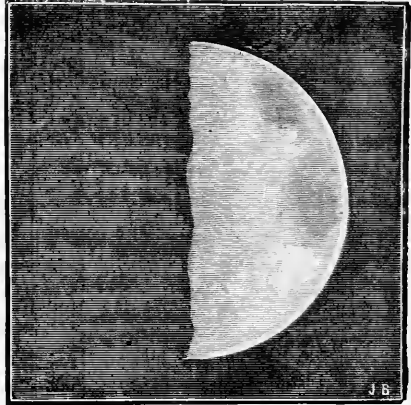
Vénus observée à la lunette (4 février 1883).
